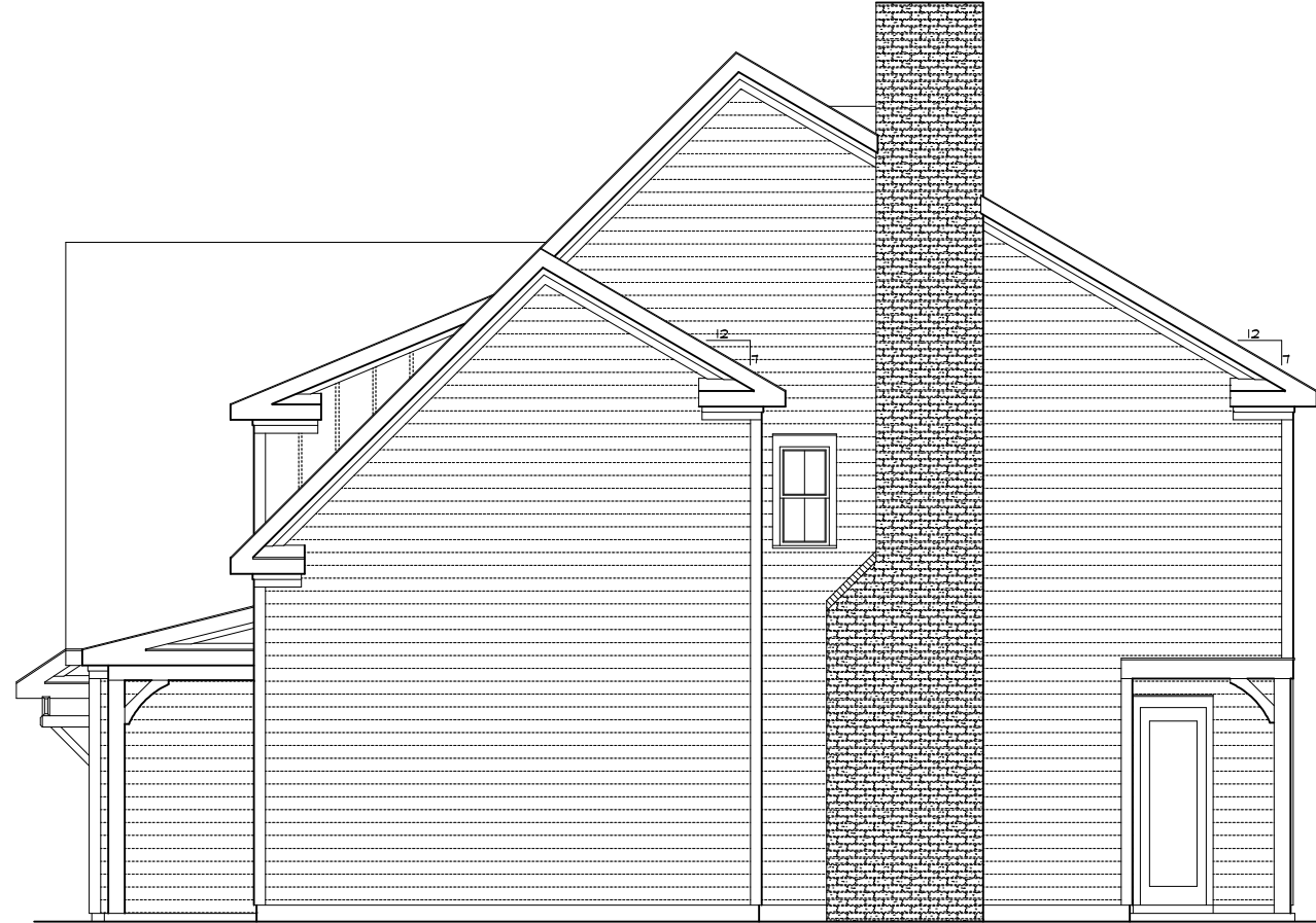
RIGHT ELEVATION
